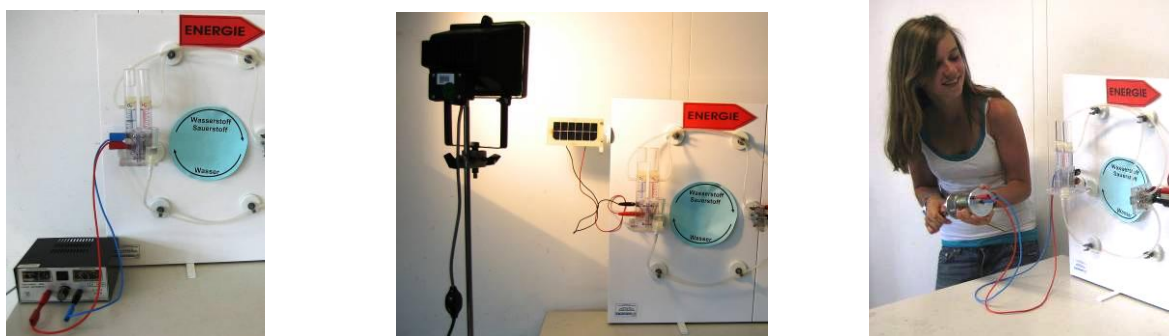
Abb. 3: Antrieb des chemischen Energie-Träger-Stromkreises mithilfe eines Netzgeräts, eines Handgenerators, einer Solarzelle
