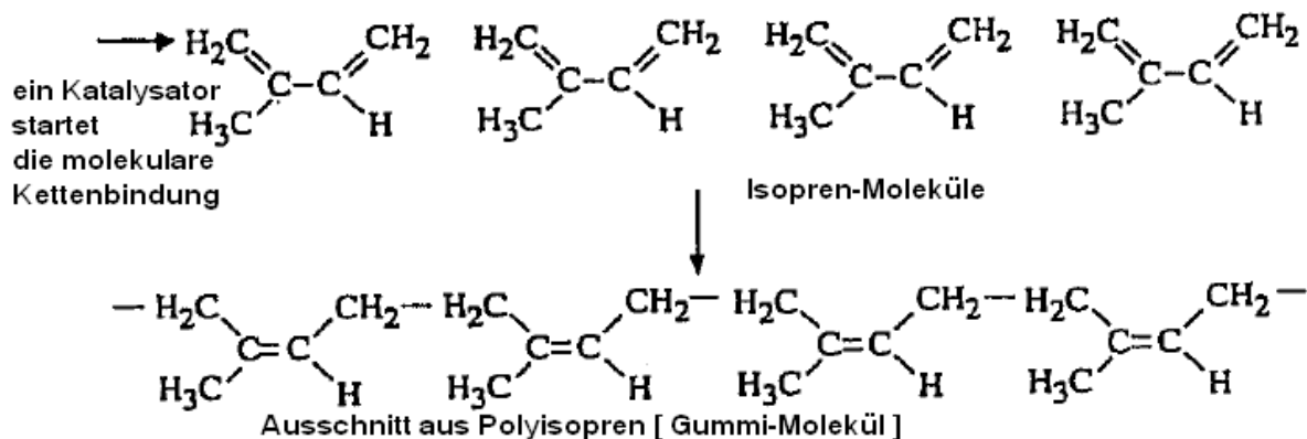
Abbildung: Ein Katalysator startet die molekulare Kettenbildung — Isopren-Moleküle — Ausschnitt aus Polyisopren, das Gummi-Molekül
